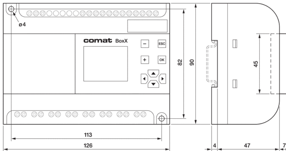
Fig. 2.4 Abmessungen AF-20
