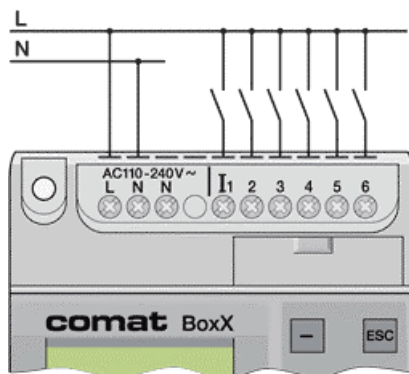
Fig. 2.7 AC Typen
