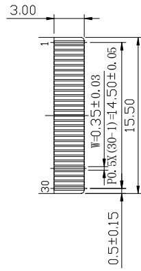
DETAIL *A* (S: 2/1,2PLS)
