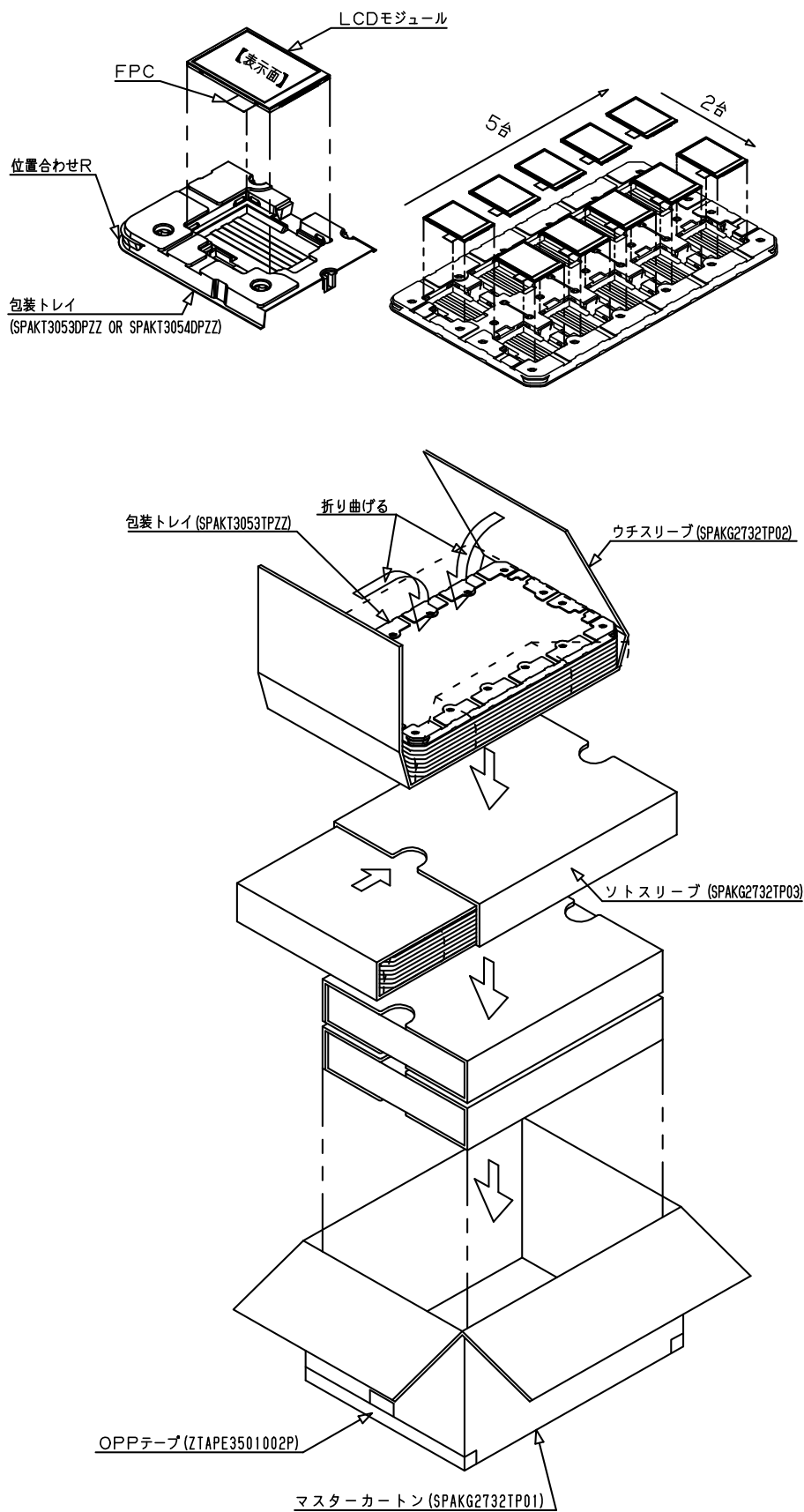
図8：包装形体図
